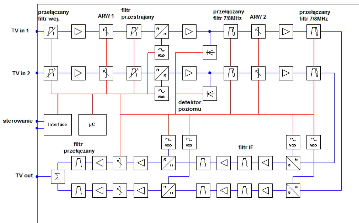
Rys. 1. Schemat blokowy podwójnego pełnopasmowego przemiennika kanałowego TV analogowej/cyfrowej typu OK 45A (WISI)
