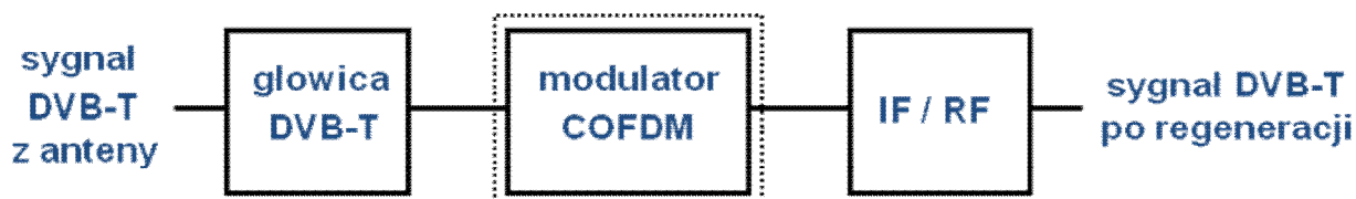
Rys. 2. Schemat blokowy regeneracji sygnału DVB-T w panelu OV 75M 4041 (WISI)
