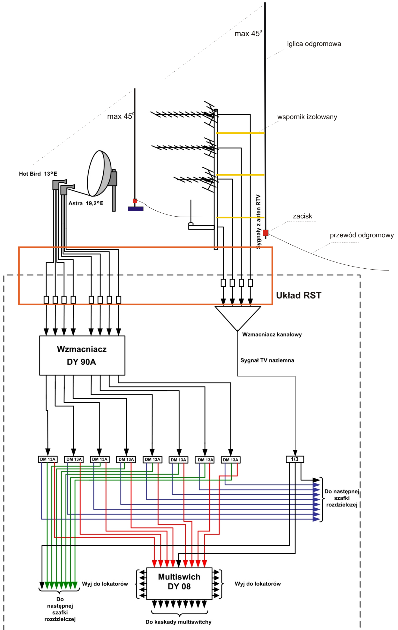
Schemat szafki rozdzielczej
